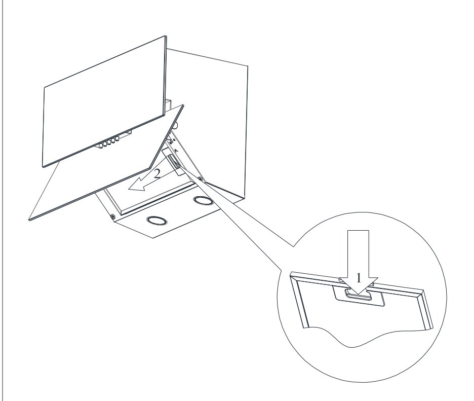
Rys. 7 Demontaż filtra aluminiowego przeciwłuszczowego.
