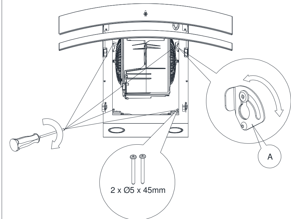
Rys. 9 Montaż osłony kominowej.
