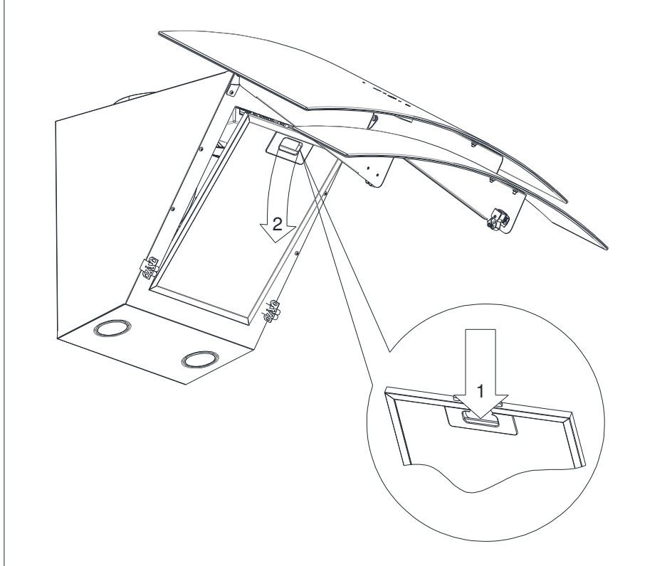
Rys. 6 Demontaż filtra aluminiowego przeciwłuszczowego.
