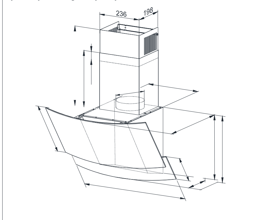
Rys.2 Rysunek gabarytowy
